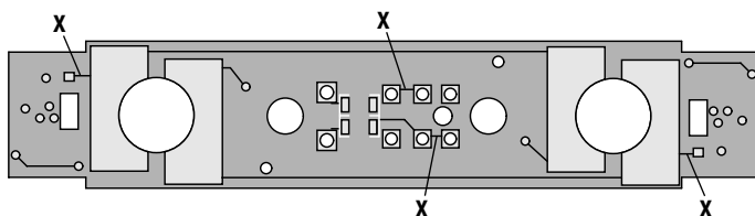
Fig. 3 Platine Unterseite/PCB lower side
